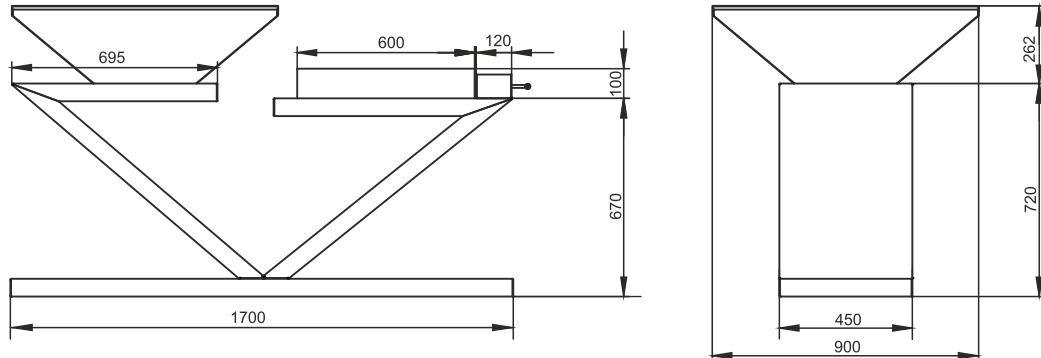
Barbecue-firepit G5
