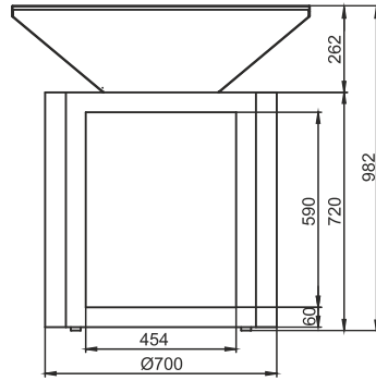
Barbecue-firepit G2
