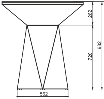
Barbecue-firepit G1
